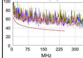
ACR-F (dB)
